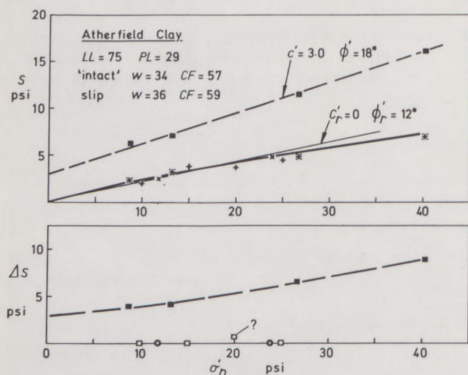
Fig. 14. Sevenoaks: test results on Atherfield Clay at Pit WB1. Sevenoaks: résultats d'essais sur l'argile d'Atterfield à la fouille WB1.
