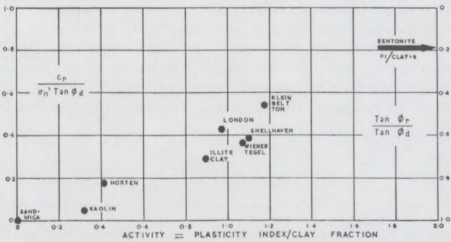
Fig. 2 Relation Between the Components of Shear Strength and the Activity of Normally Consolidated Clays Relation entre les composantes de la résistance au cisaillement et l'activité d'argiles normalement consolidés
