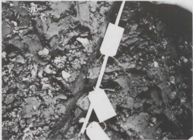
Fig. 30. Wraysbury: sampling at a joint in the London Clay. Wraysbury: échantillonnage d'un joint dans le London Clay.
