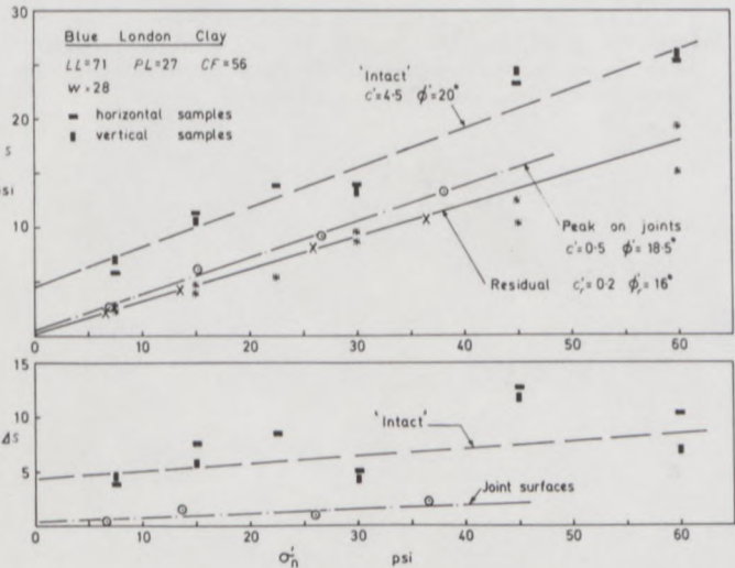
Fig. 31. Wraysbury: test results on joint surfaces. Wraysbury: résultats d'essais.
