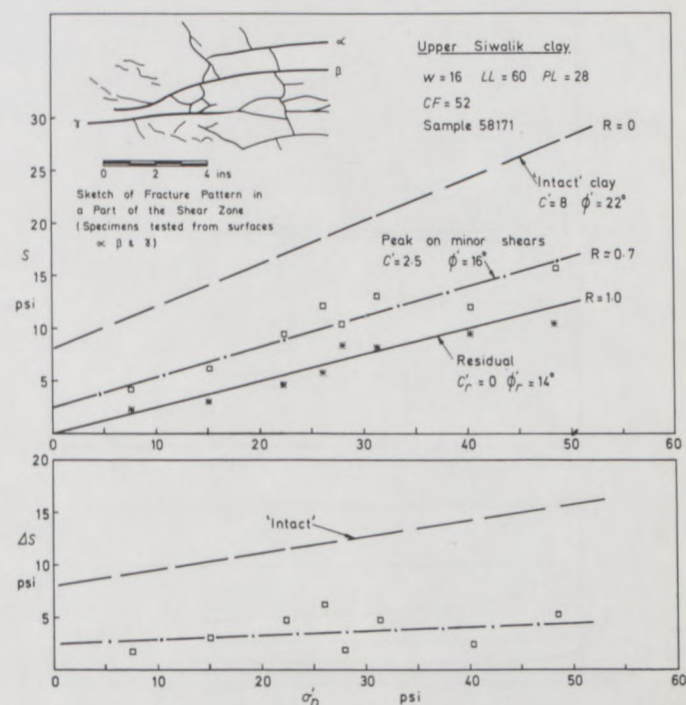
Fig. 27. Mangla: test results on minor shears in shear zone Bed 512 at Sukian. Mangla: résultats d'essais sur des discontinuités secondaires au Lit 512 à Sukian.
