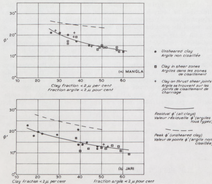
Fig. 4 Correlations between Residual Angle of Friction and Clay Fraction for Clay Bedrock at Mangla and Jari. Corrélation entre l'angle de frottement résiduel et la fraction argile pour l'assise en argile à Mangla et à Jari.
