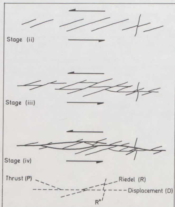
Fig. 1. Successive stages in the development of a shear zone in clay, from laboratory tests (Skempton 1966). Etapas successives dans le développement d'une zone de cisaillement dans l'argile, d'après des essais au laboratoire. (Skempton 1966).
