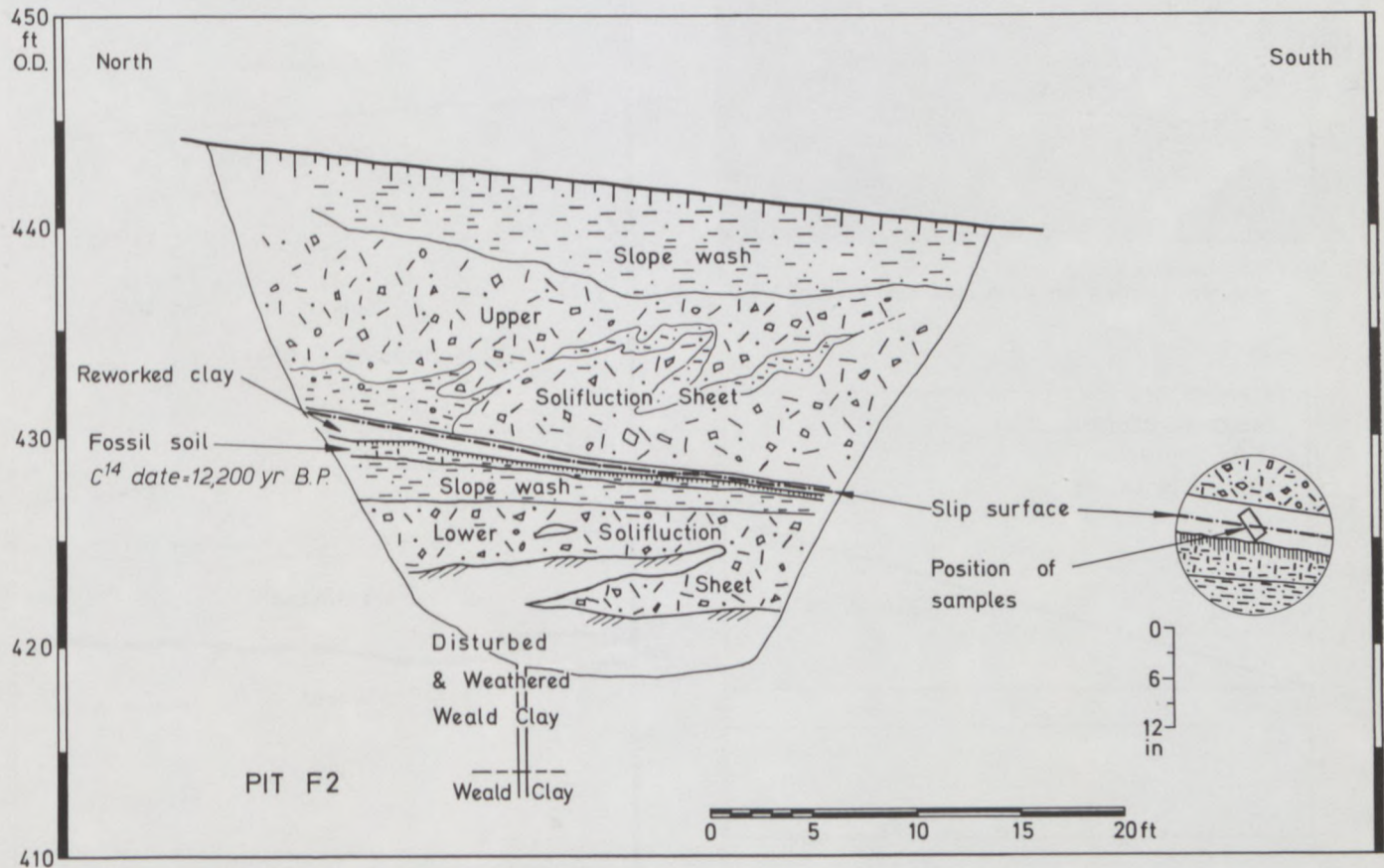
Fig. 16. Sevenoaks : section through upper and lower solifluction sheets at Pit F2. Sevenoaks : coupe des nappes supérieures et inférieures de solifluxion à la fouille F2.
