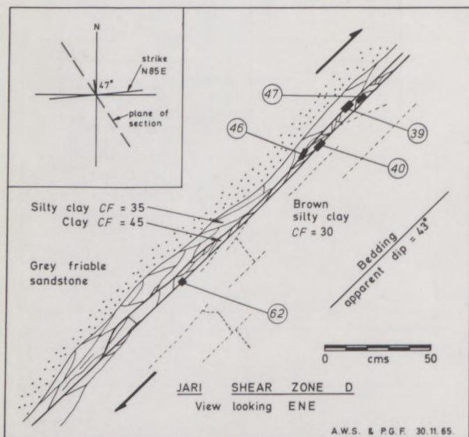
Fig. 24. Mangla: shear zone D at Jari. Mangla: zone de cisaillement D à Jari.
