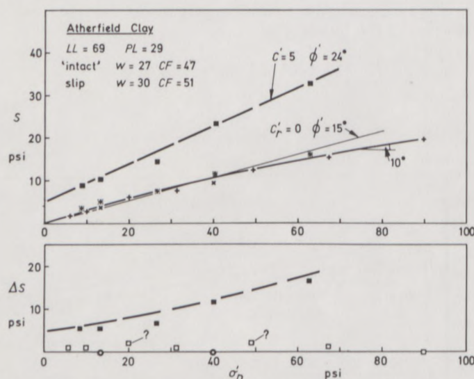
Fig. 15. Sevenoaks: test results on Atherfield Clay at Pit WB2. Sevenoaks: résultats d'essais sur l'argile d'Atterfield à la fouille WB2.
