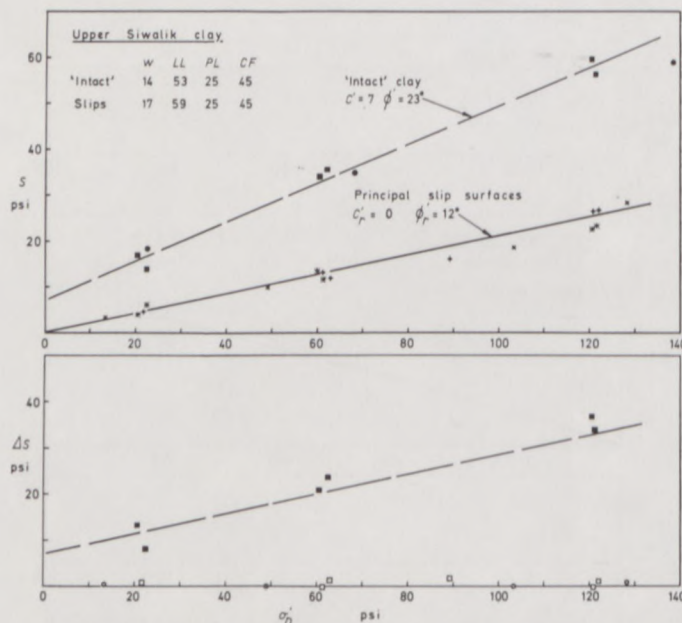
Fig. 25. Mangla: test results on shear zone D at Jari. Mangla: résultats d'essais sur la zone de cisaillement D à Jari.
